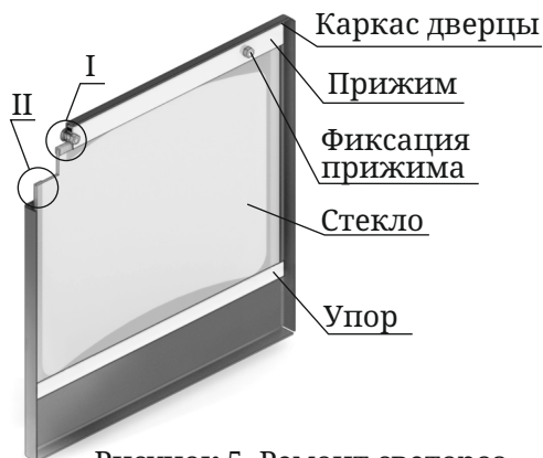
Рисунок 5. Ремонт светорозрачного экрана дверцы
