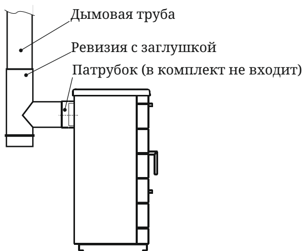
Рисунок 4. Схема присоединения печи к дымоходу
