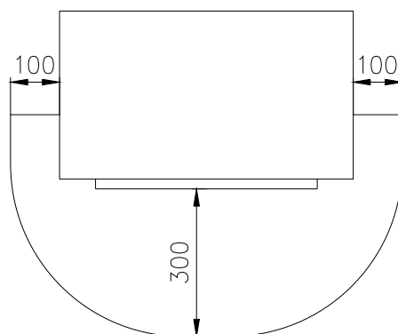
Прокладка рис.2
