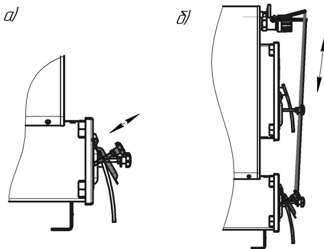
Рисунок 9 — Регулировка подачи воздуха
