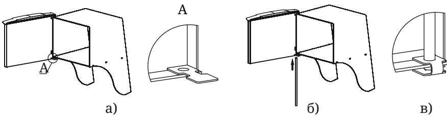
Рисунок 5. Установка дверцы при монтаже печи
