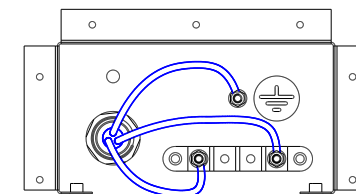
Рис.3.1 Подключение
