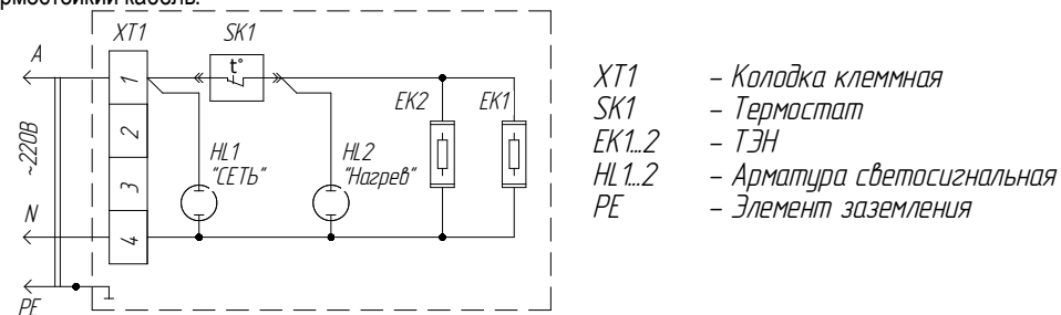
Рис.3 Схема электрическая принципиальная
