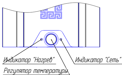
Рис.5 Органы управления
